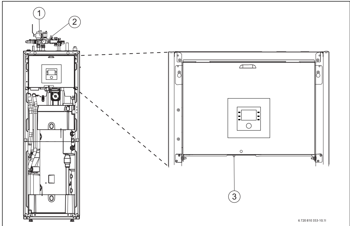
sl. 6 Unutrašnja jedinica AWM / AWMS
