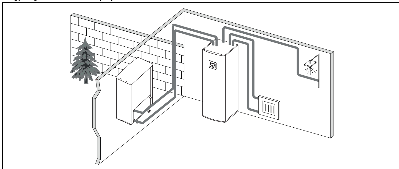
sl. 3 Toplotna pumpa Compress 6000 AW, unutrašnja jedinica AWM / AWMS sa integrisanim bojlerom za toplu vodu i električnim dogrevačem
