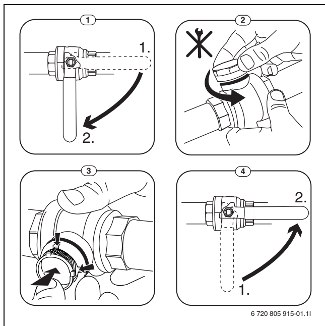
sl. 7 Čišćenje sita
