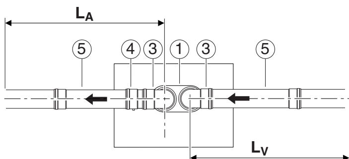
sl. 11 Vođenje izduvnih gasova po C 12
