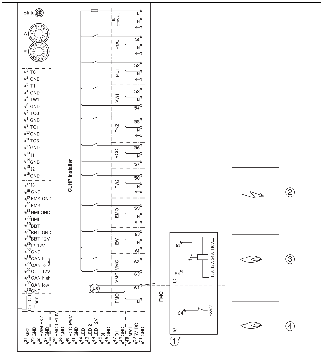
sl. 37 Priključna šema za instalacioni modul, alarm eksternog dogrevača
