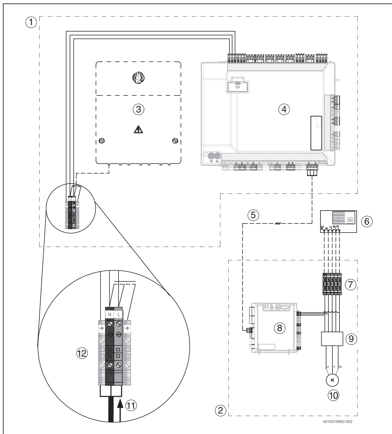
sl. 34 Trofazna toplotna pumpa i unutrašnja jedinica sa eksternim dogrevačem
