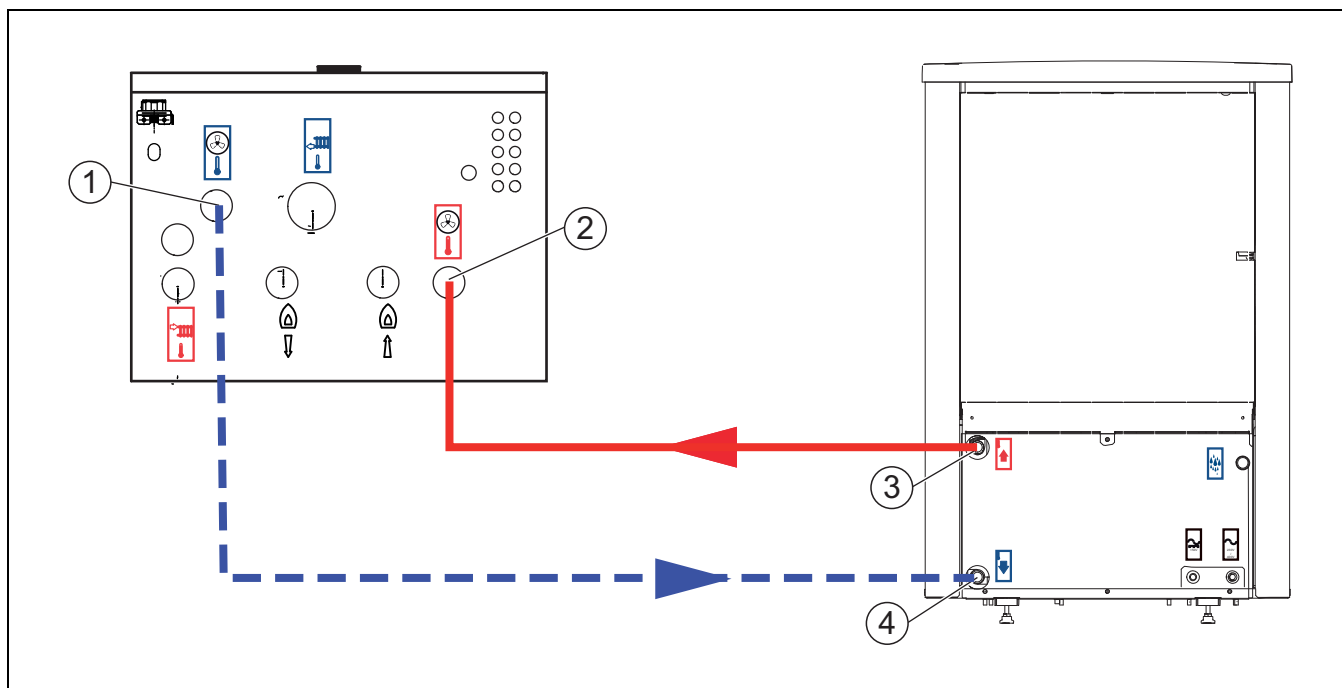
sl. 6 Priključak unutrašnje jedinice na toplotnu pumpu
