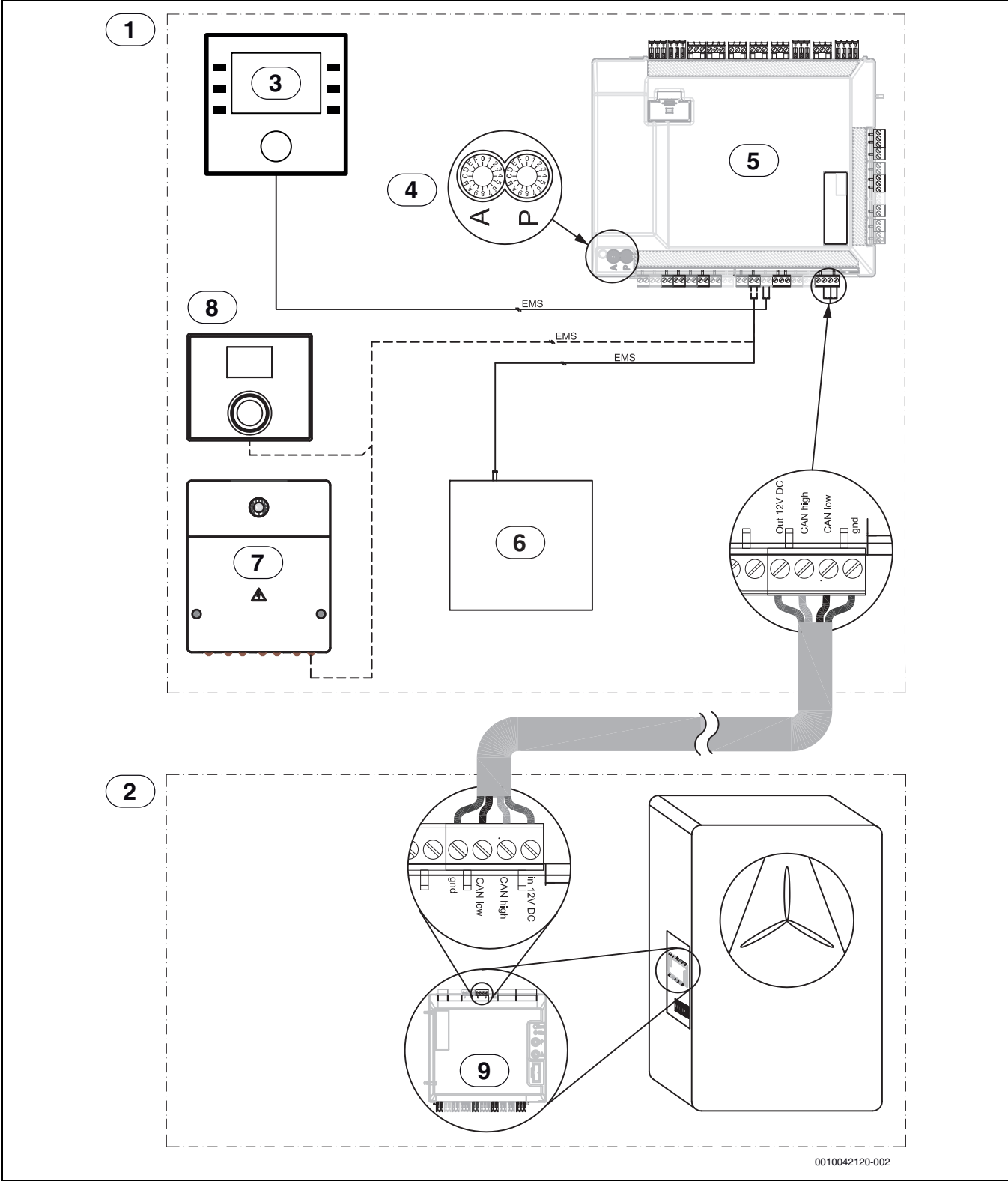
sl. 32 Unutrašnja jedinica sa mešačem za eksterni dogrevač – pregled CAN/EMS-BUS
