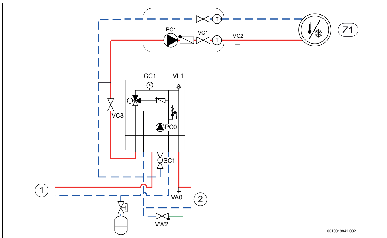
sl. 8 Unutrašnja jedinica sa eksternim dogrevačem i sistemom grejanja
