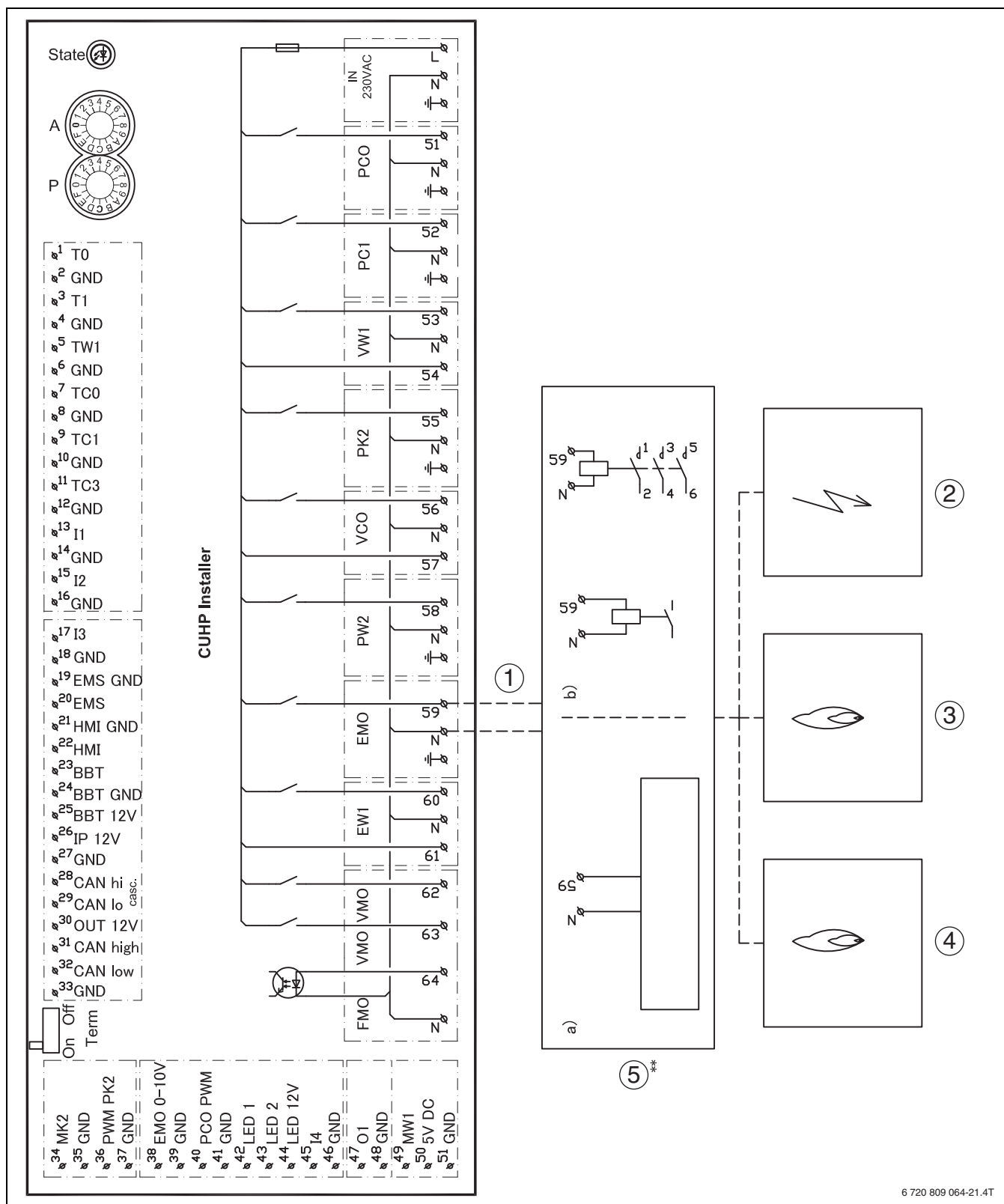
sl. 36 Priključna šema za instalacioni modul, start/stop sa eksternim dogrevačem
