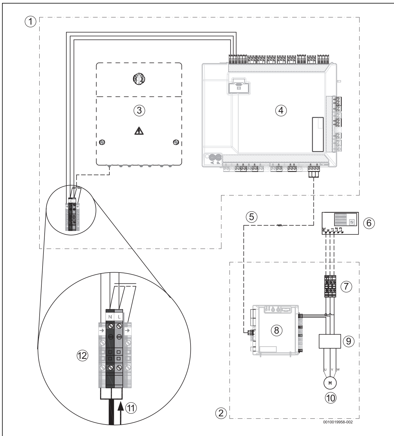
sl. 33 Jednofazna toplotna pumpa i unutrašnja jedinica sa eksternim dogrevačem
