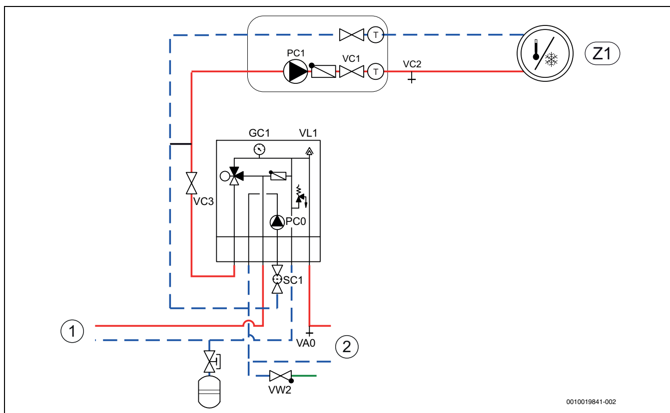
sl. 19 Unutrašnja jedinica sa eksternim dogrevačem i sistemom grejanja
