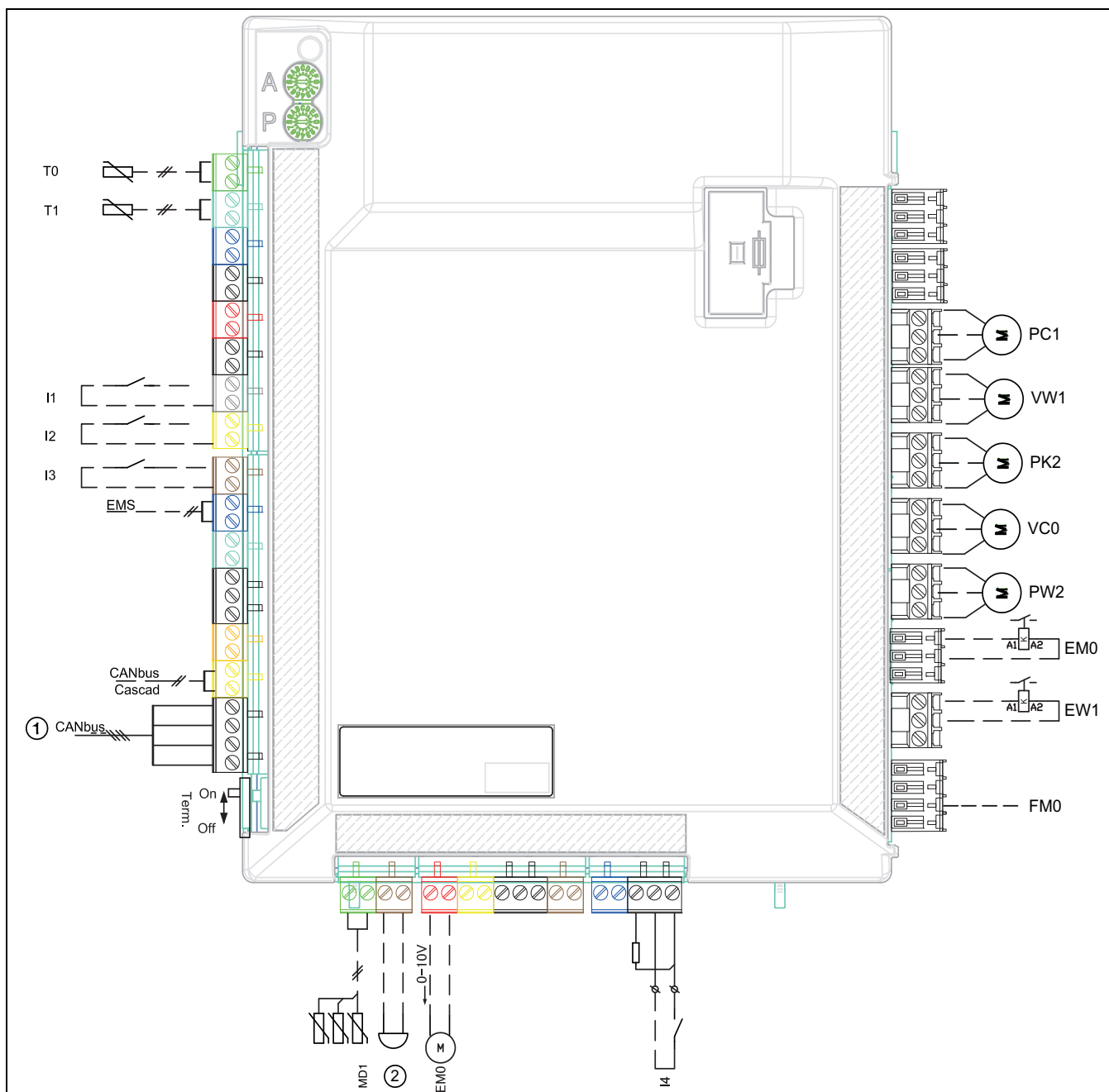
sl. 12 Priključci instalacionog modula
