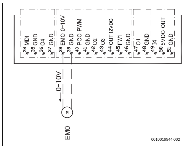
sl. 13 Regulacioni signal od 0 do 10 V za eksterni dogrevač
