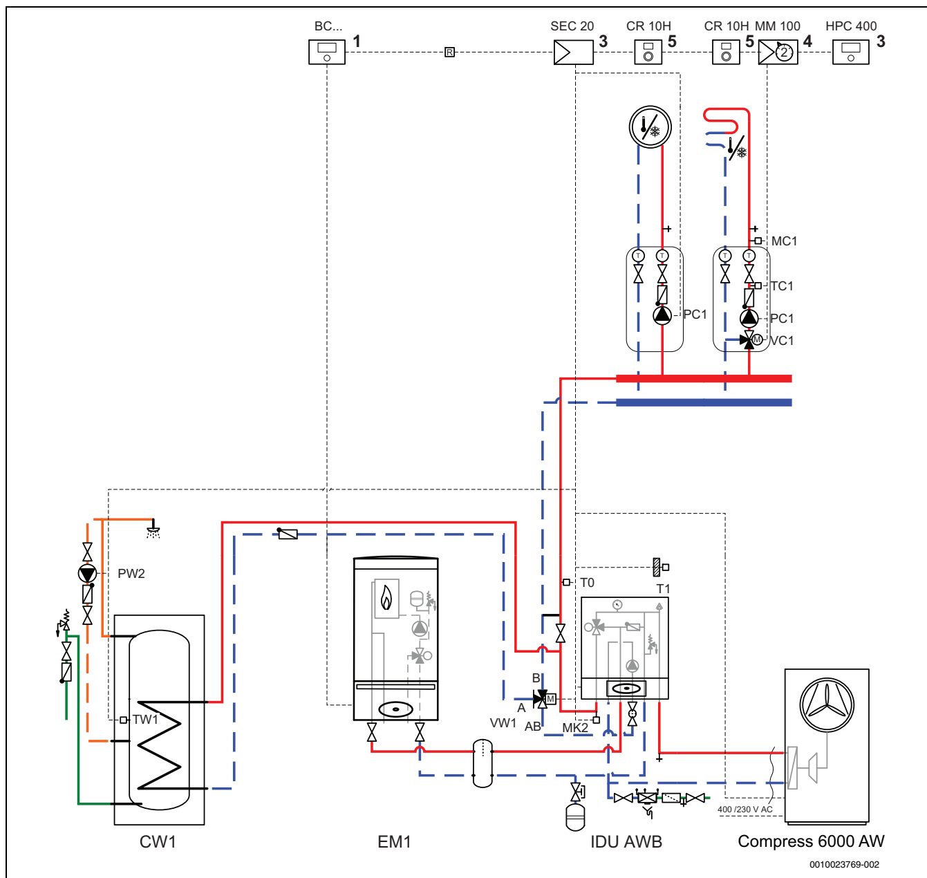
sl. 31 Dogrevač sa mešačem sa bojlerom za toplu vodu
