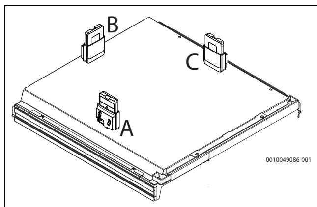
sl. 16 Pričvršćivanje držača na gornji poklopac unutrašnje jedinice. Pored držača, slika prikazuje i Connect-Key koji se nalazi u držaču
