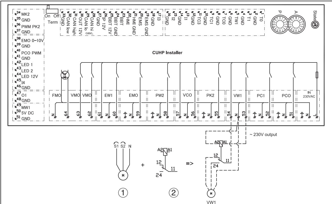
sl. 38 Alternativna instalacija 3-krakog prebacivačkog ventila
