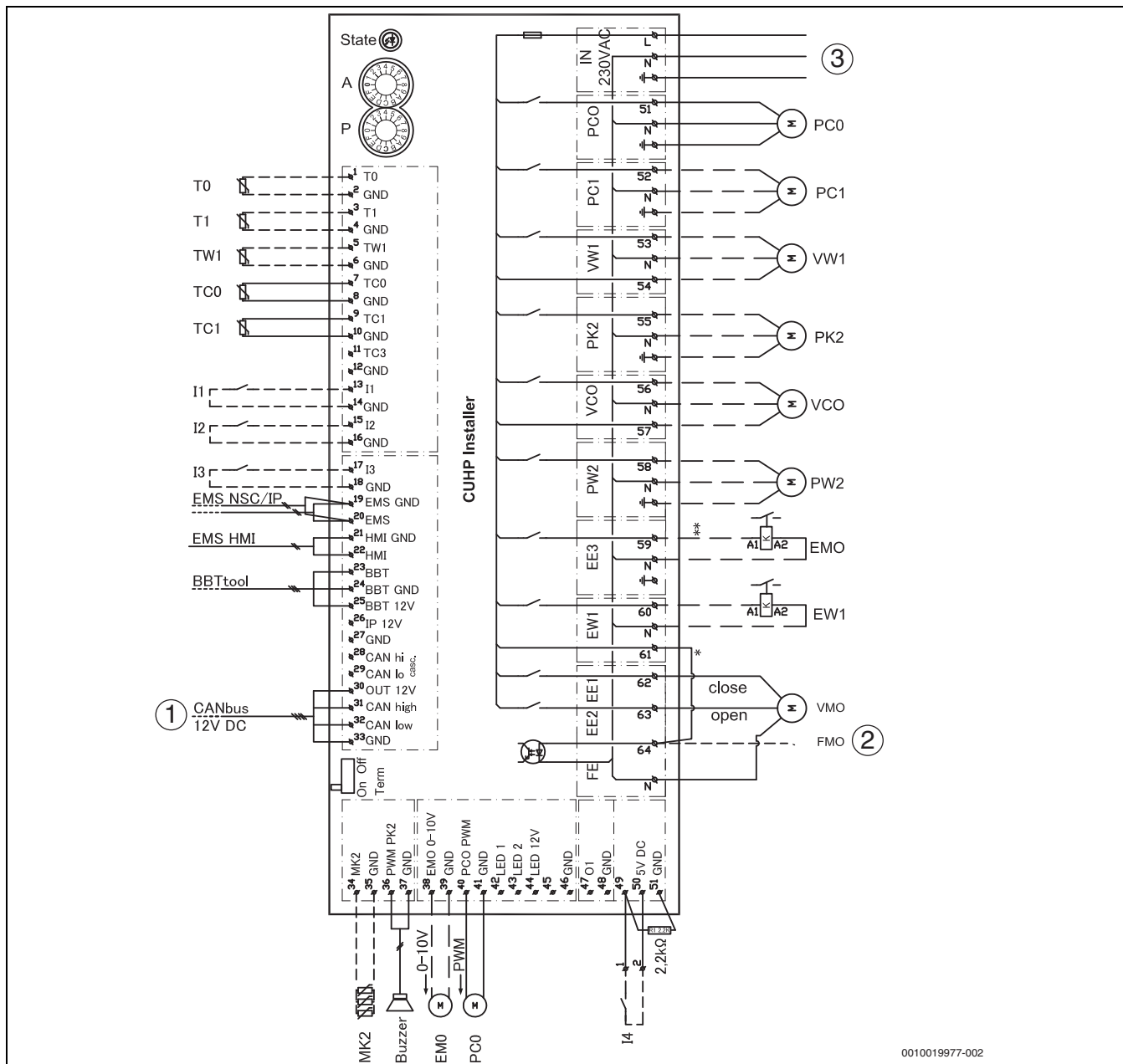
sl. 35 Priključna šema instalacionog modula za unutrašnju jedinicu sa mešačem za eksterni dogrevač
