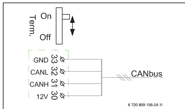
sl. 9 Terminacija CAN-BUS-a
