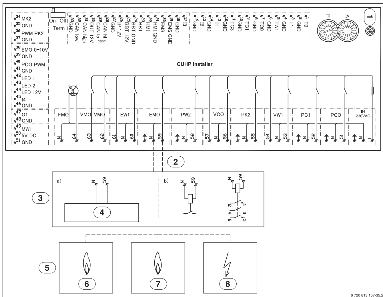
sl. 13 Šema veze instalacionog modula, uključivanje/isključivanje
