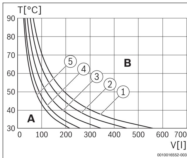
sl. 11 Karakteristike ekspanzione posude
