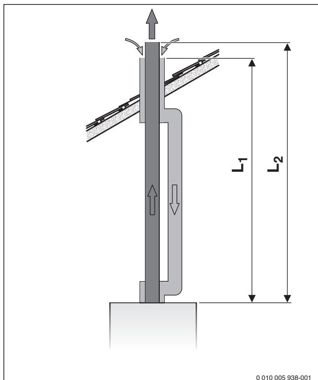
sl. 9 Vertikalni odvod izduvnih gasova sa razdvojnjom cevi C 32
