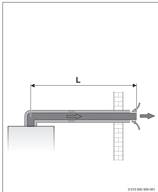
sl. 6 Horizontalni odvod za izduvne gasove c koncentričnom cevi C 12
