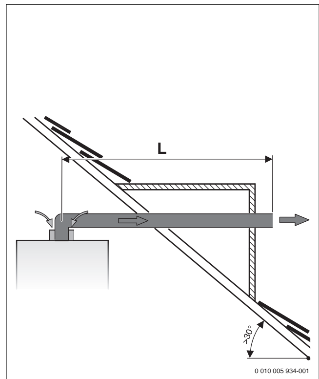
sl. 4 Horizontalni odvod izduvnih gasova B 22
