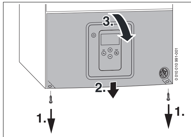
sl. 14 Otvaranje upravljačkog uređaja nadole
