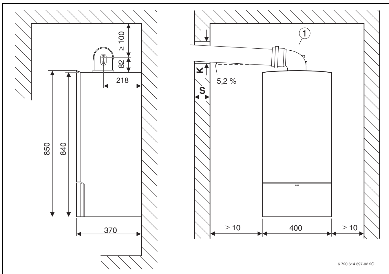
sl. 6 Dimovod Ø 60/100 mm
