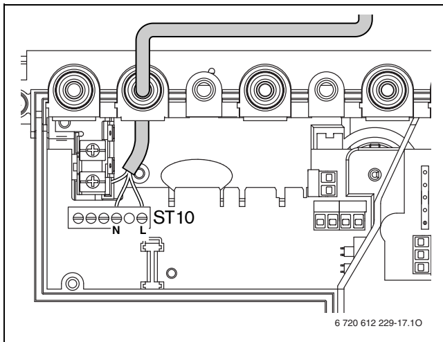
sl. 29 Terminalna traka za snabdevanje naponom ST10
