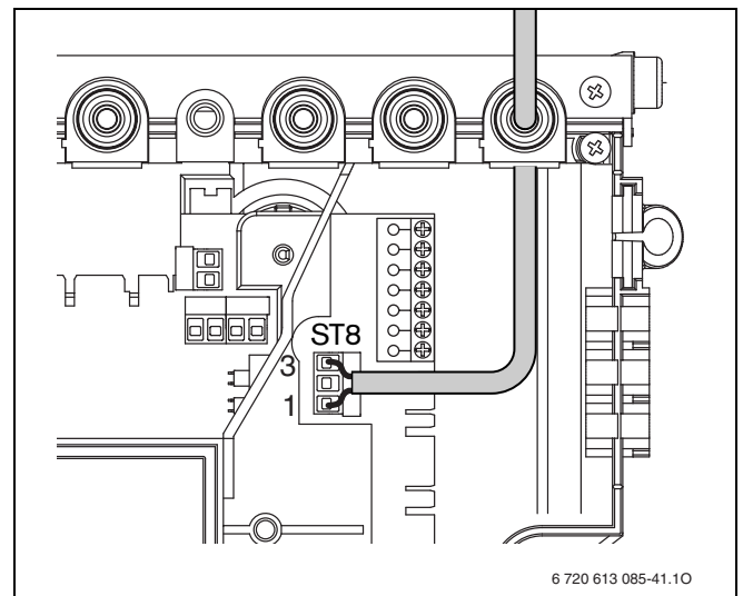
sl. 26 Priključak termostata bojlera
