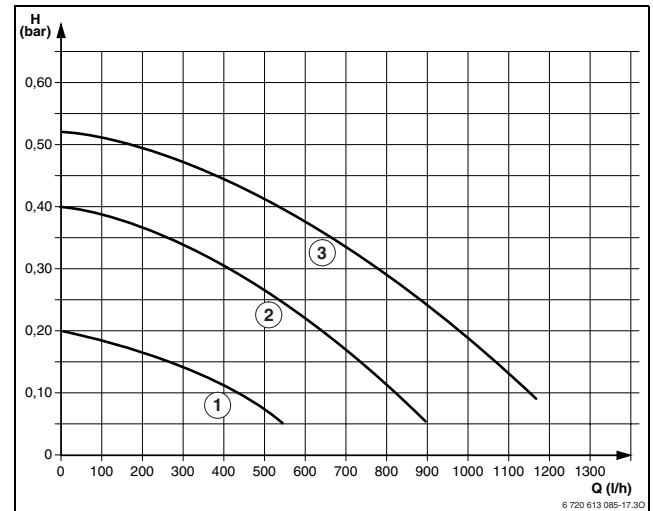
sl. 40 Karakteristike pumpe kod ZSC 24-3, ZWC 24-3 (bez montažne priključne ploče)
