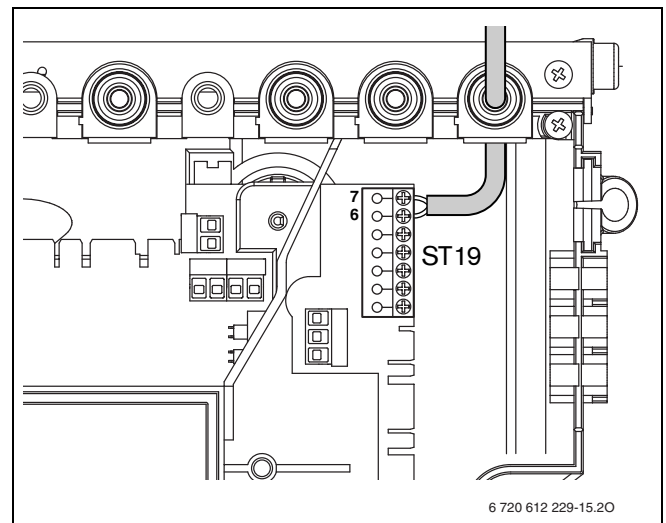
sl. 19 Priključak regulatora
