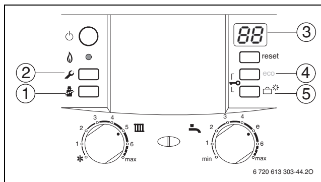
sl. 44 Pregled elemenata upravljanja
