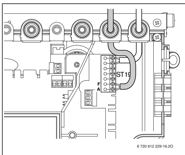
sl. 20 Priključak spoljnog senzora
